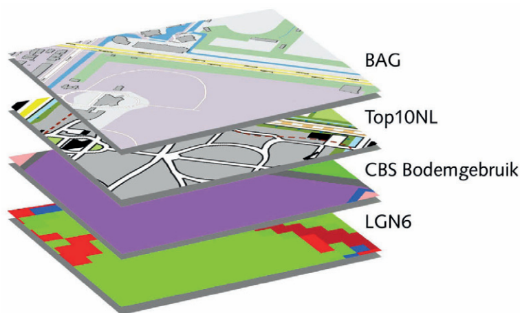
FIGUUR 3.2 DOOR HET SLIM SAMENVOEGEN VAN DE VERSCHILLENDE KAARTEN WORDT EEN BETERE LANDGEBRUIKKAART GEMAAKT DAN DOOR DE KAARTEN AFZONDERLIJK
